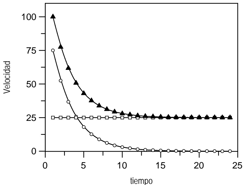
Figura 5. Efecto de la optimización de una proteína sobre su velocidad de evolución. La velocidad de evolución de una proteína ( \sigma ) es la suma de la velocidad de evolución de la parte funcional ( \circ ) y la no funcional ( \square ). Al principio, cuando la proteína está poco optimizada, su parte funcional evoluciona muy deprisa, y esta velocidad va disminuyendo hasta llegar a ser nula cuando se alcanza la estructura óptima. Por el contrario, la velocidad en la zona no funcional es independiente del grado de optimización de la proteína, por lo que es siempre constante.
